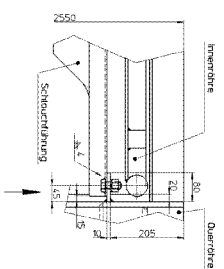
Einzelheit X
