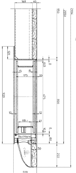
Schnitt A-A
